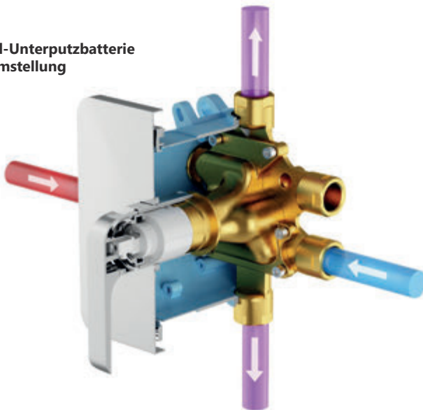
Einhand-Unterputzbatterie mit Umstellung
