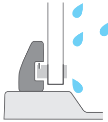
Duschabtrennung mit Rahmen 10°, Pivot, Blix Slim, Blix, Objekt
